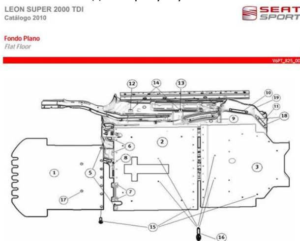
Рис. 7.3. Плоское дно.
