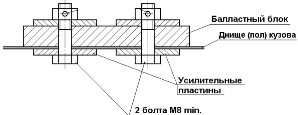
Рис. 5.2. Крепление балласта.
