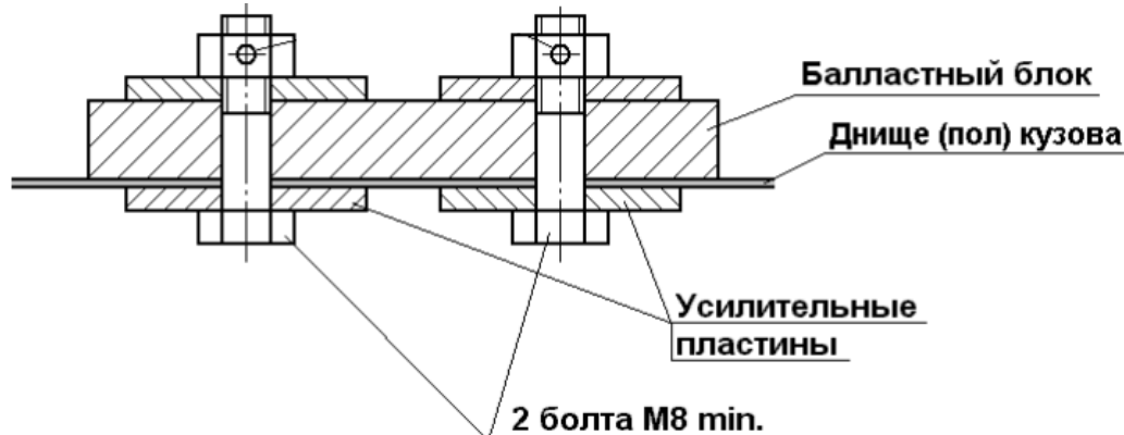
Рис. 5.2. Крепление балласта.
