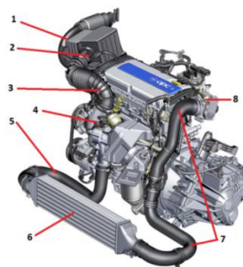
Рис. 1. Элементы системы впуска двигателя с турбонаддувом:
