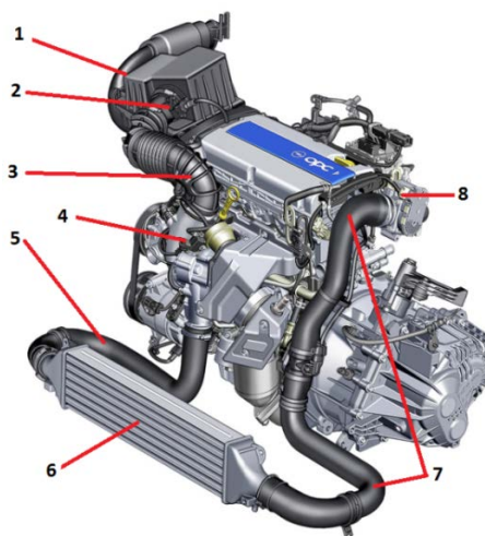
Рис. 1. Элементы системы впуска двигателя с турбонаддувом:
